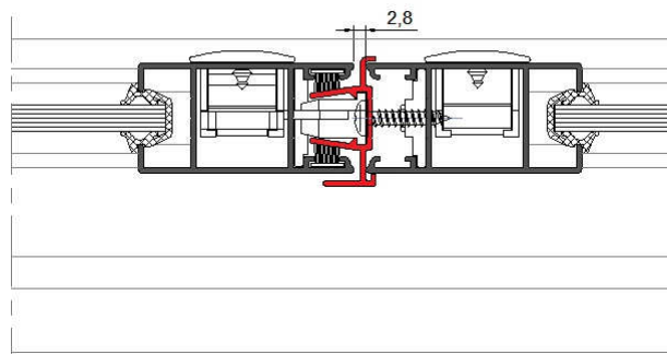
Fechamento central
