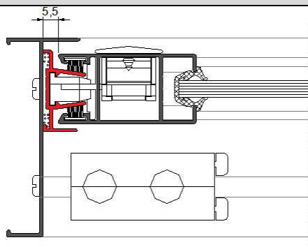
Fechamento lateral
